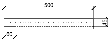
Alzado lateral (tapa final)
